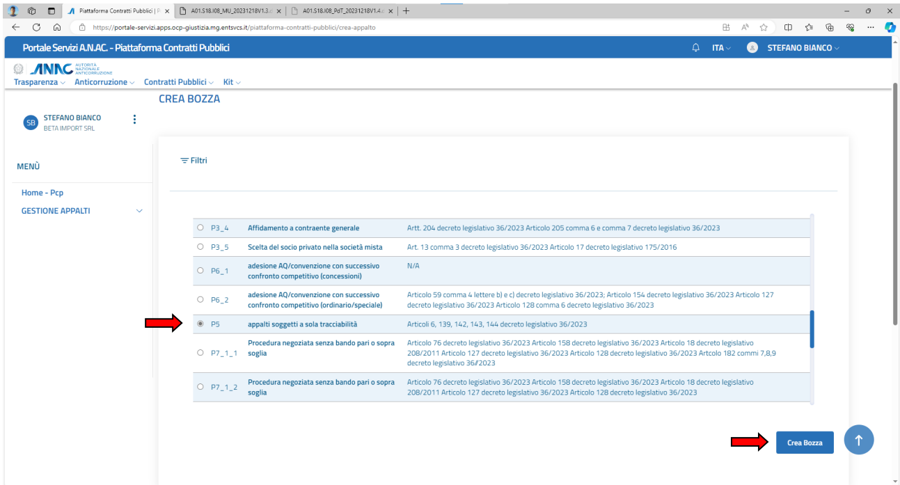
Figura 8 – crea bozza
