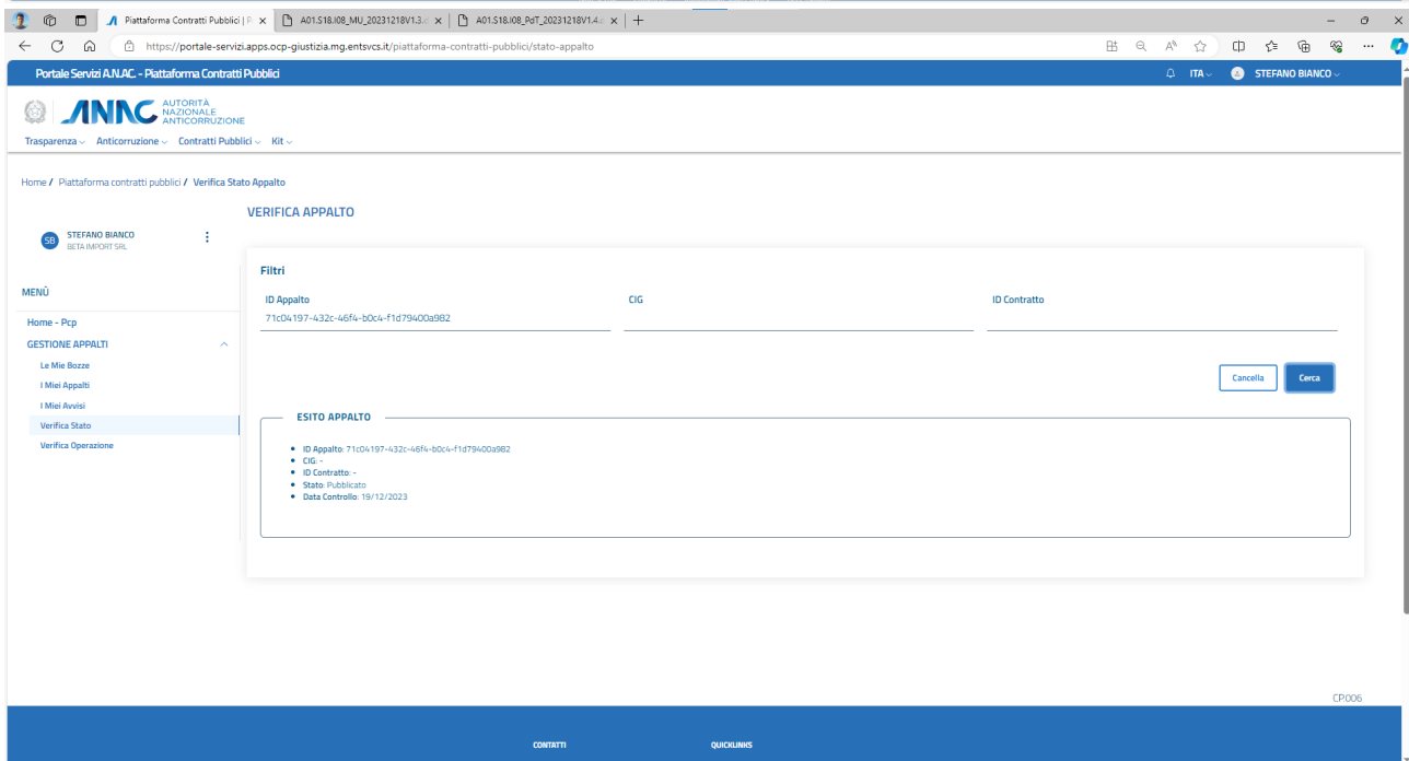
Figura 23– esito appalto
