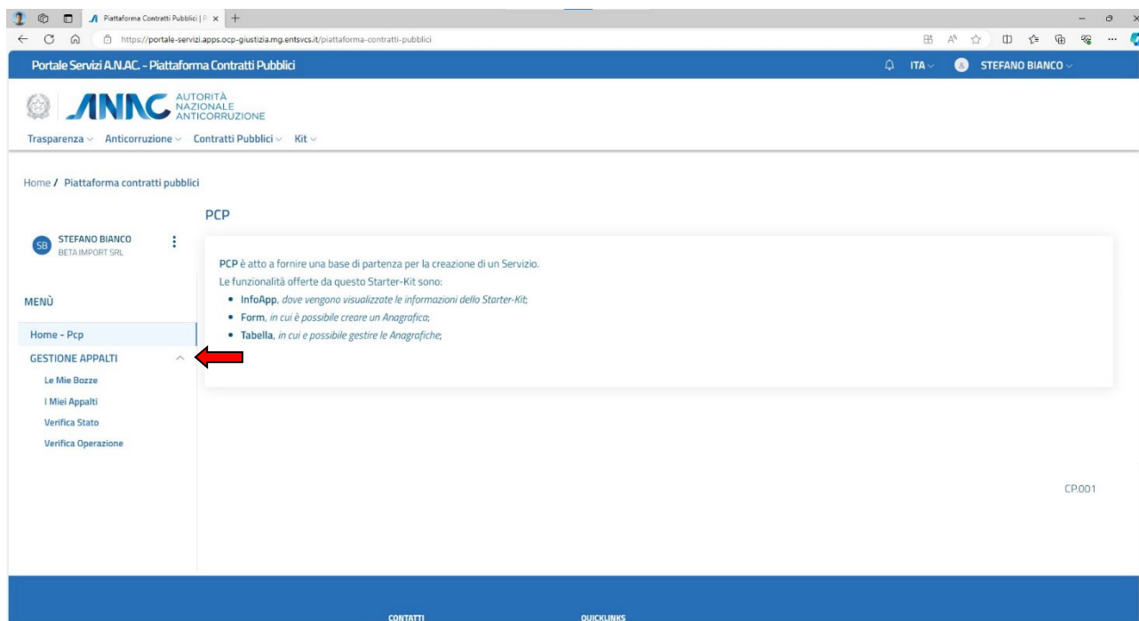
Figura 6 – menù contestuale
